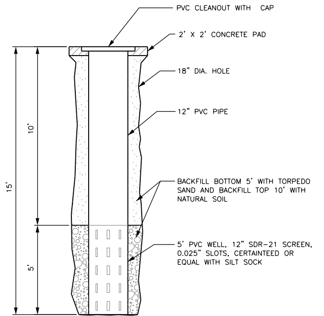
DEWATERING WELL DETAIL N.T.S.
