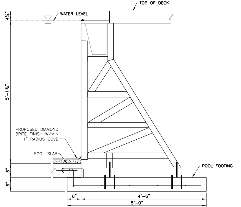
WALL SECTION DETAIL N.T.S.
